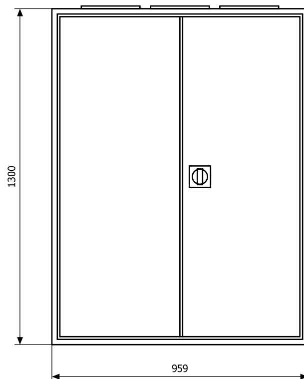
Widok elewacji
