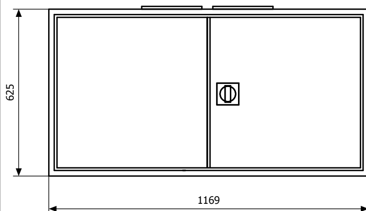
Widok elewacji
