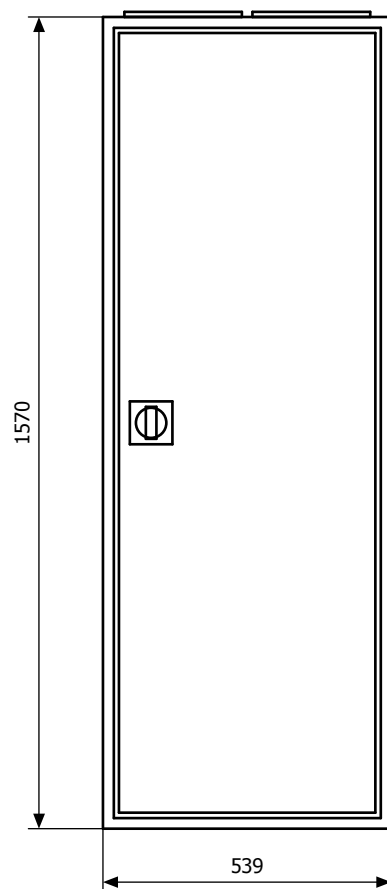
Widok elewacji
