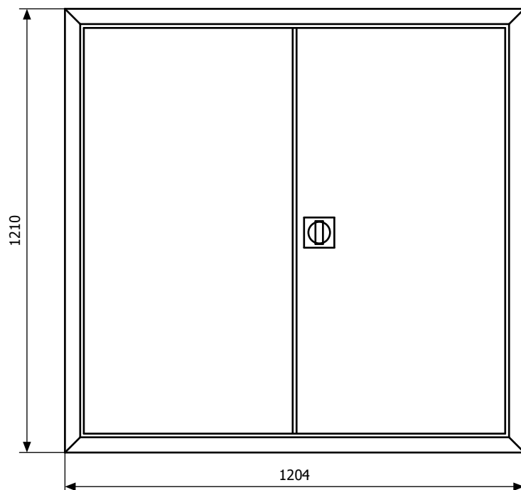
Widok elewacji
