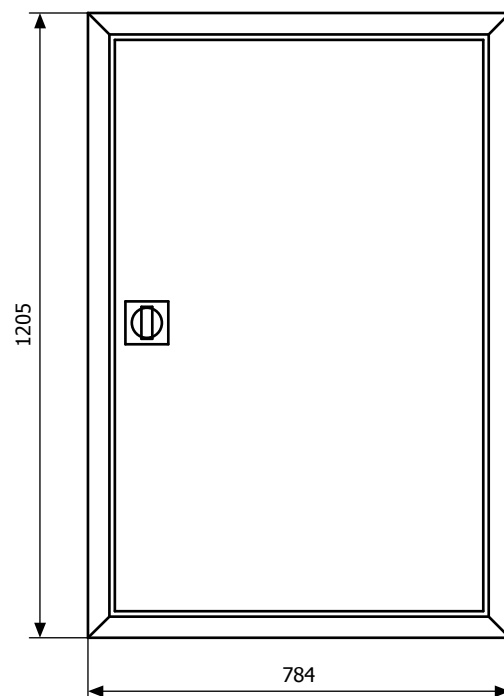
Widok elewacji
