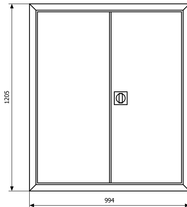
Widok elewacji
