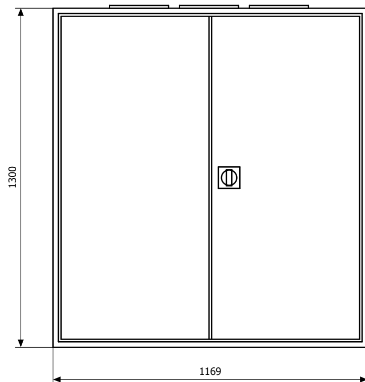
Widok elewacji
