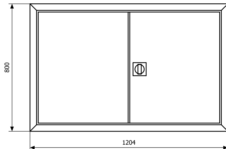
Widok elewacji
