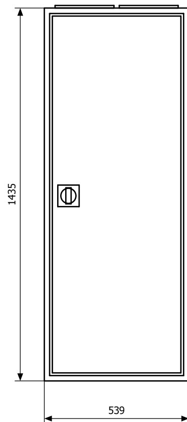
Widok elewacji
