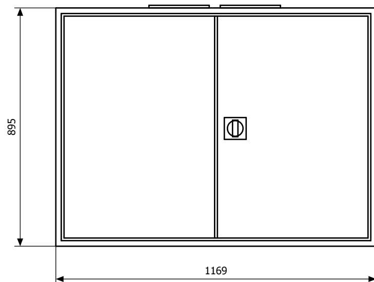
Widok elewacji
