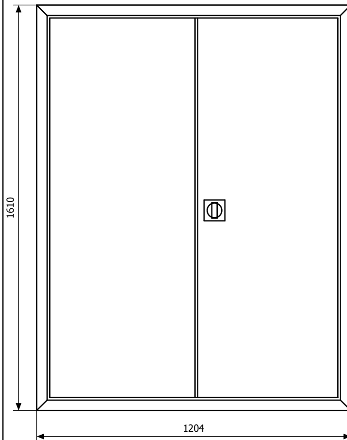
Widok elewacji
