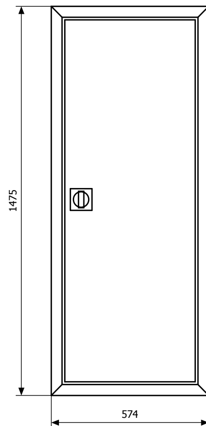
Widok elewacji
