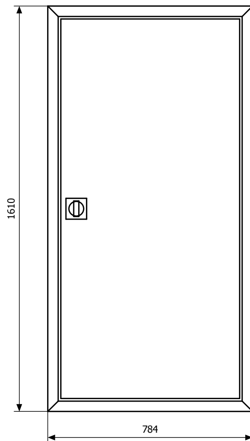
Widok elewacji
