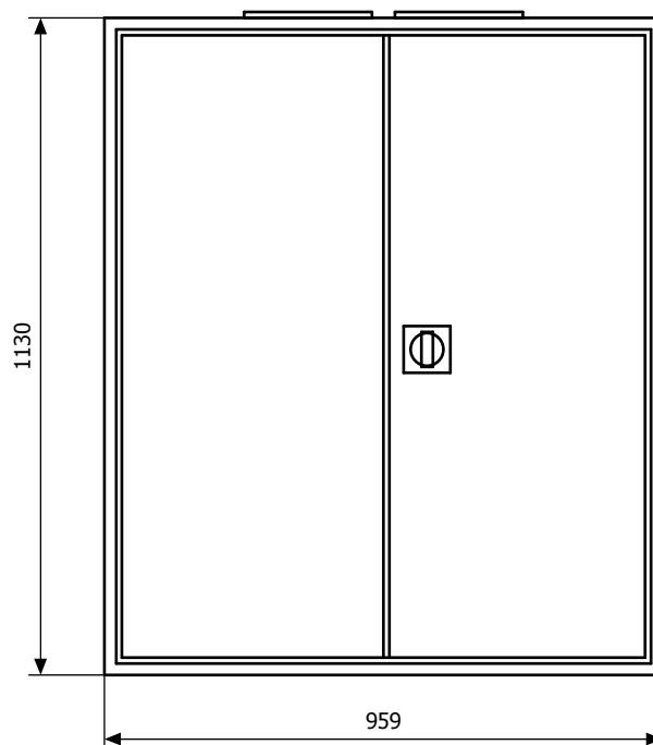
Widok elewacji
