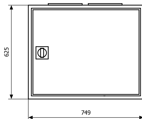
Widok elewacji
