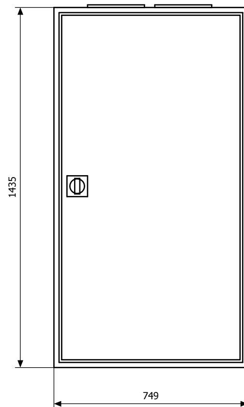
Widok elewacji
