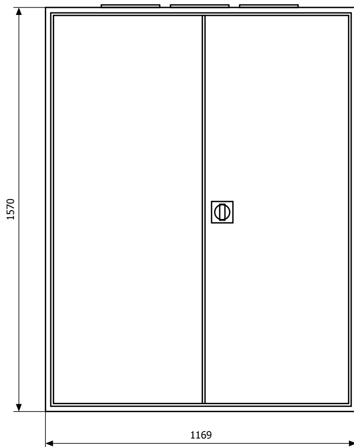
Widok elewacji
