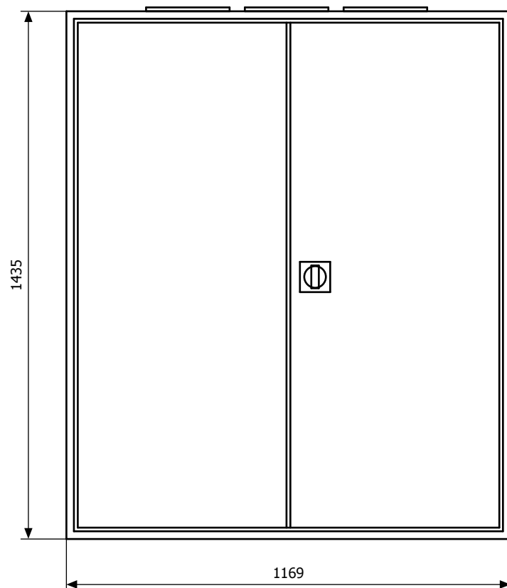
Widok elewacji
