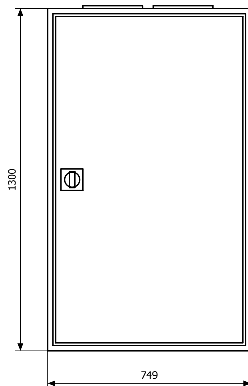
Widok elewacji
