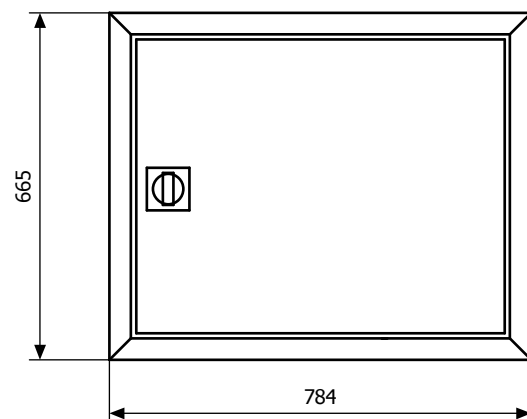
Widok elewacji
