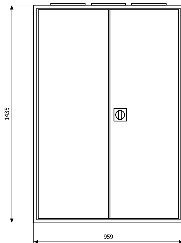
Widok elewacji
