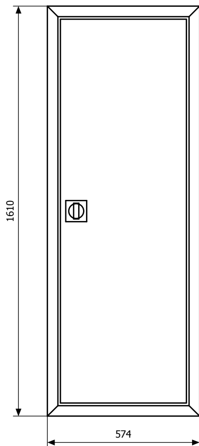
Widok elewacji
