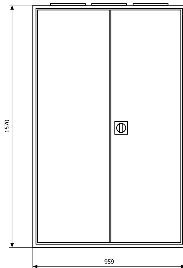
Widok elewacji
