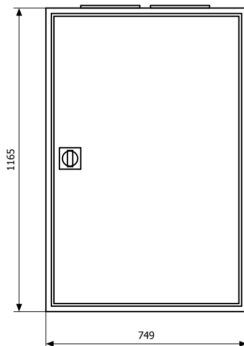
Widok elewacji
