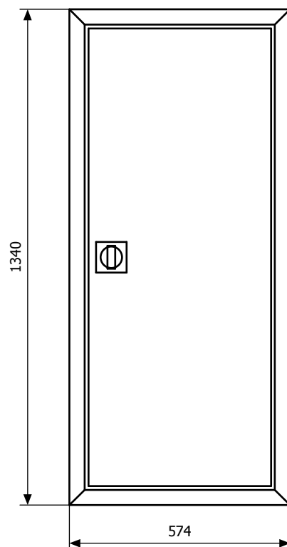
Widok elewacji
