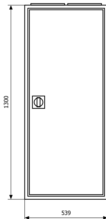
Widok elewacji
