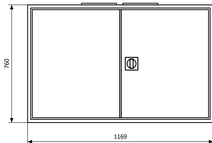
Widok elewacji
