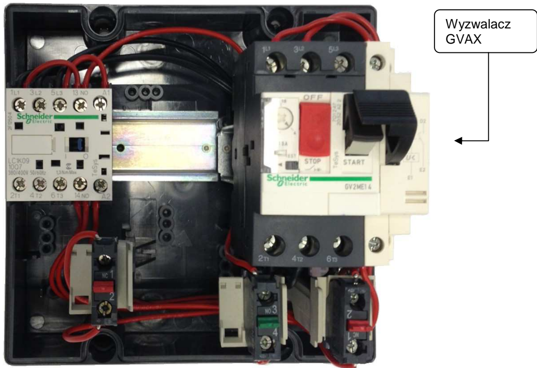
Otwarty układ rozruchowy wyposażony w GVAX385
