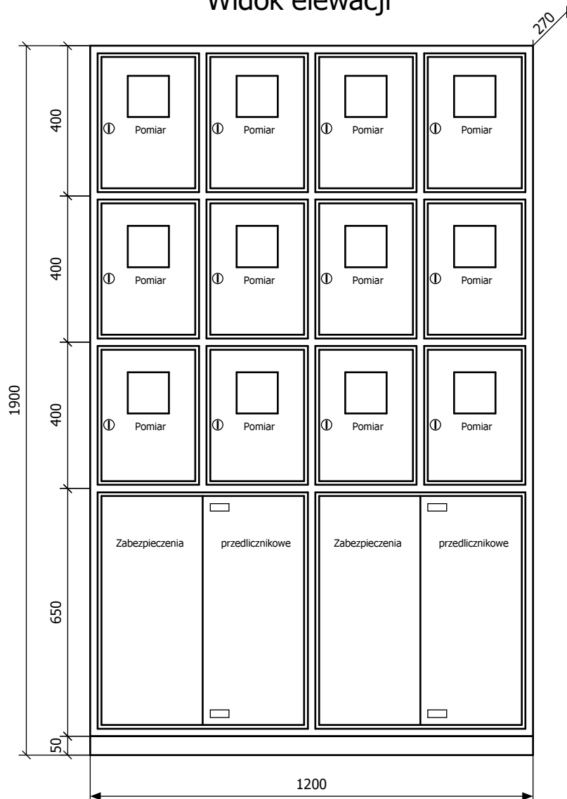
Widok elewacji
