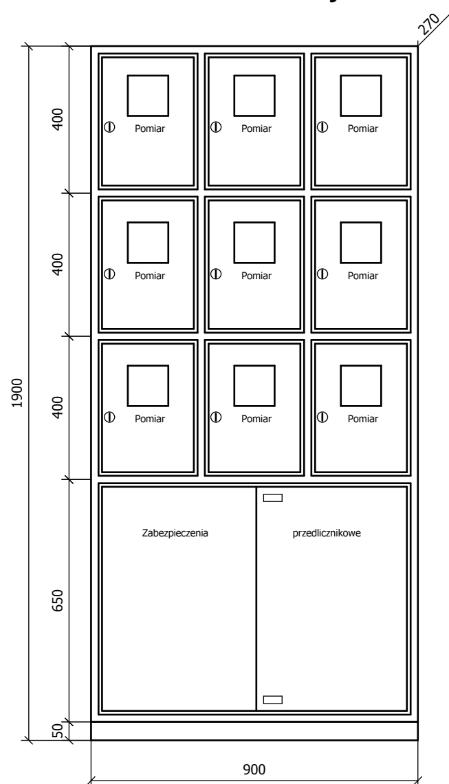
Widok elewacji
