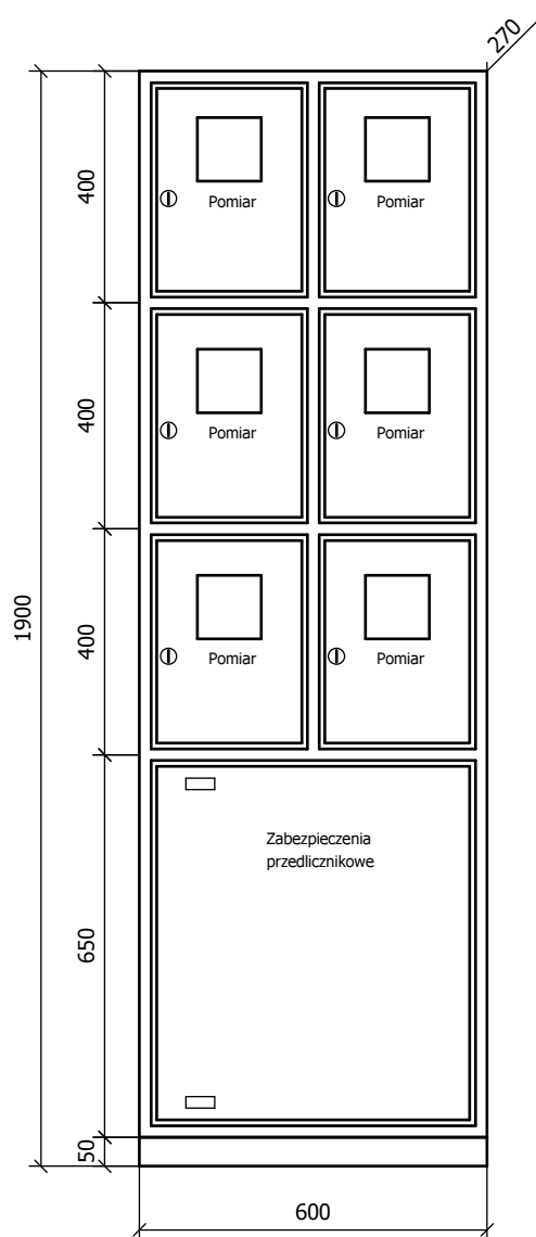
Widok elewacji
