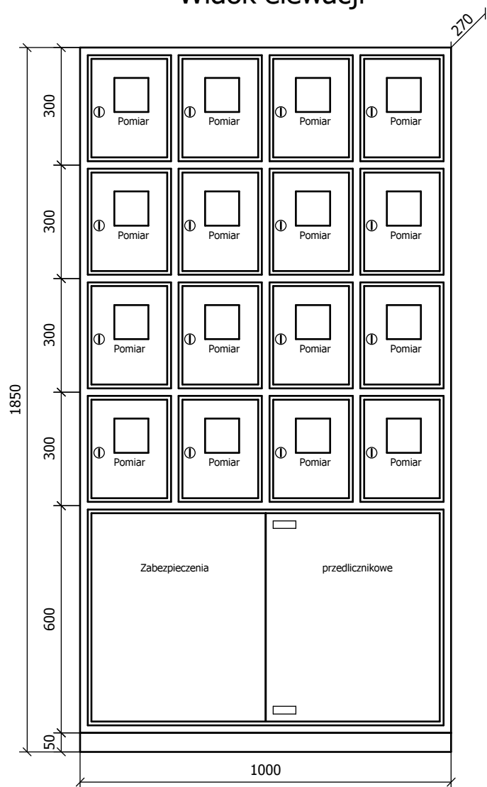
Widok elewacji
