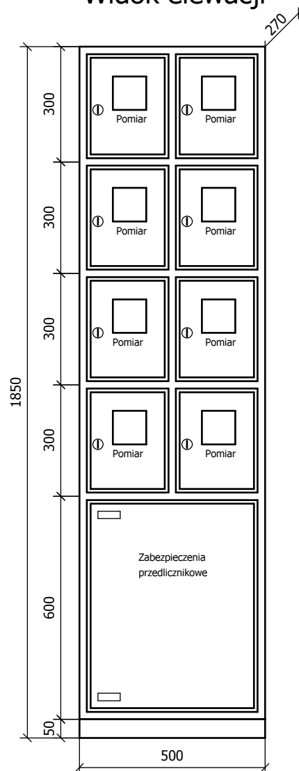
Widok elewacji
