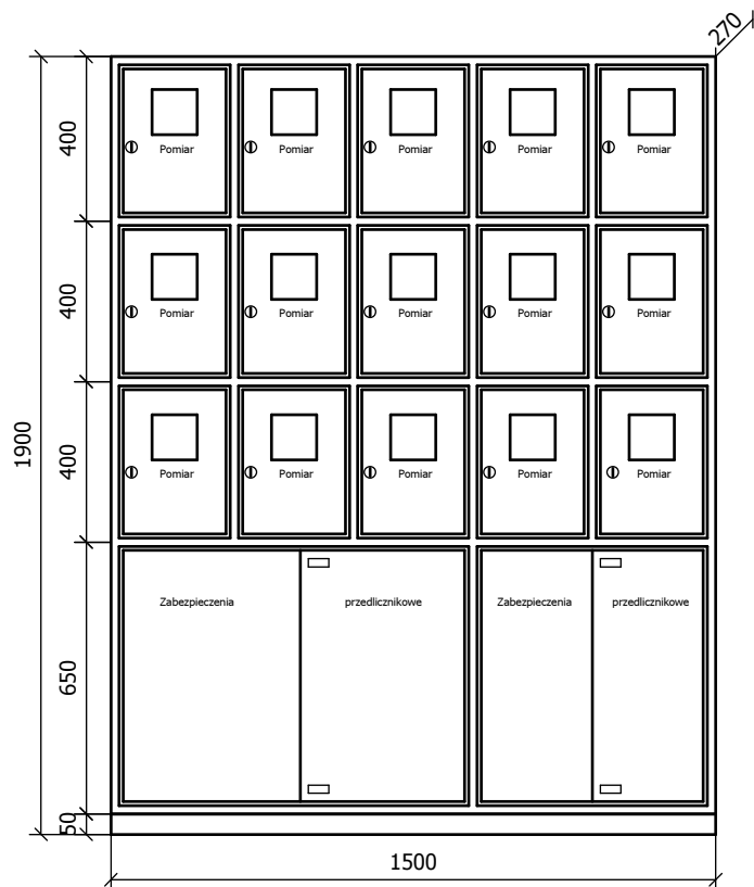
Widok elewacji
