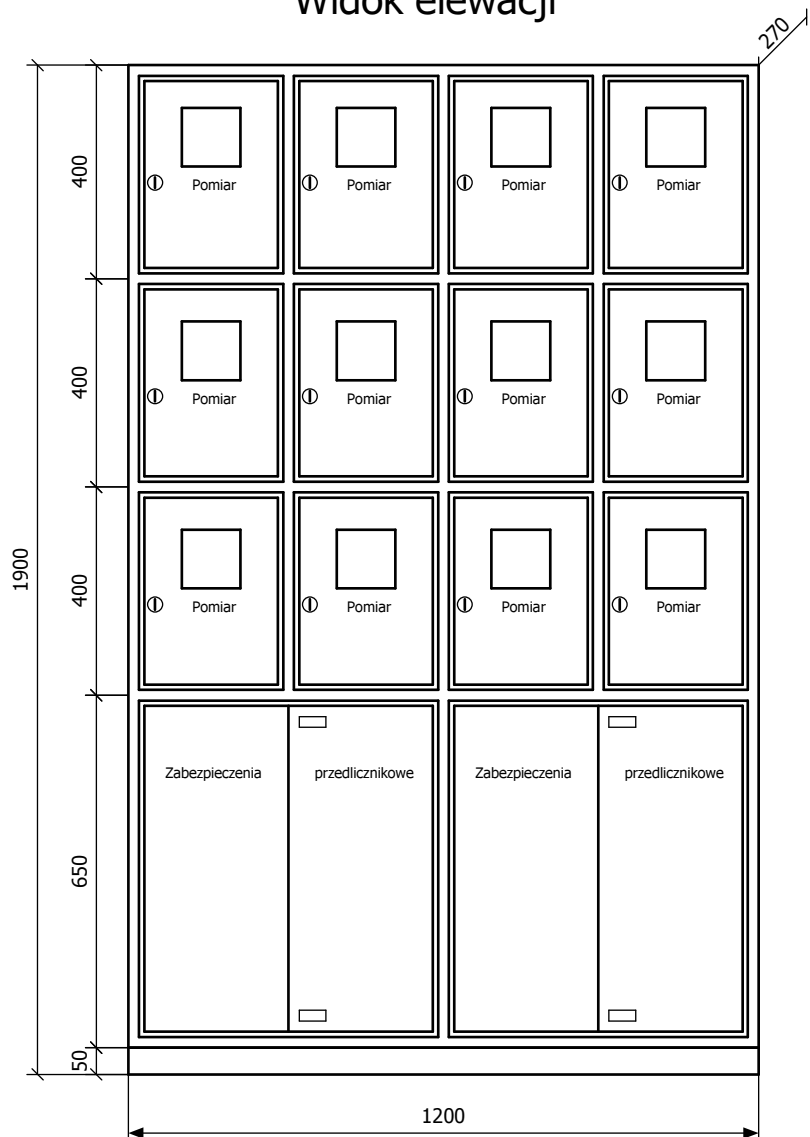
Widok elewacji
