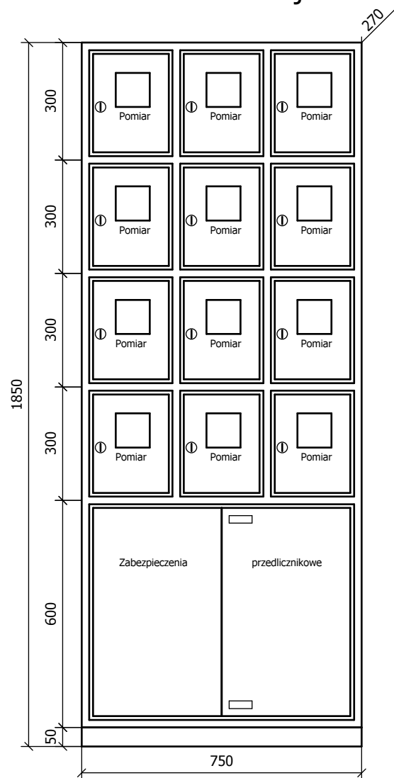
Widok elewacji
