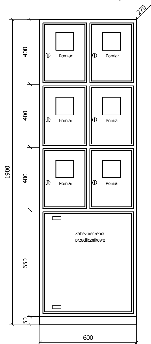
Widok elewacji
