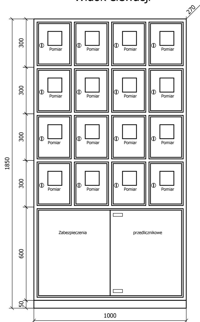
Widok elewacji
