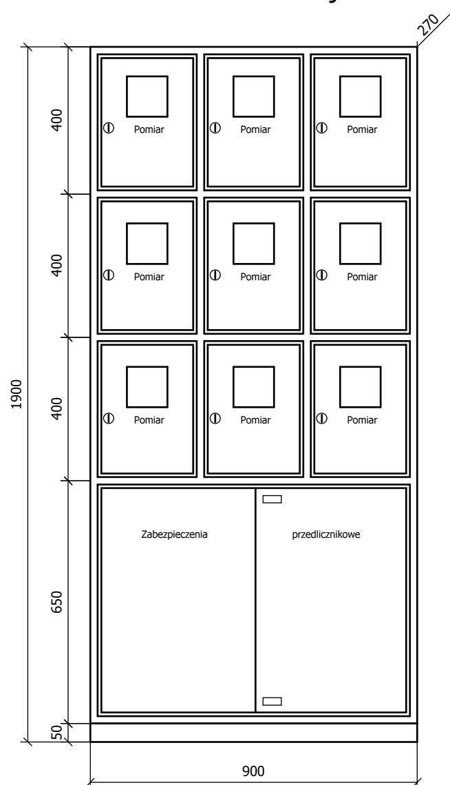
Widok elewacji
