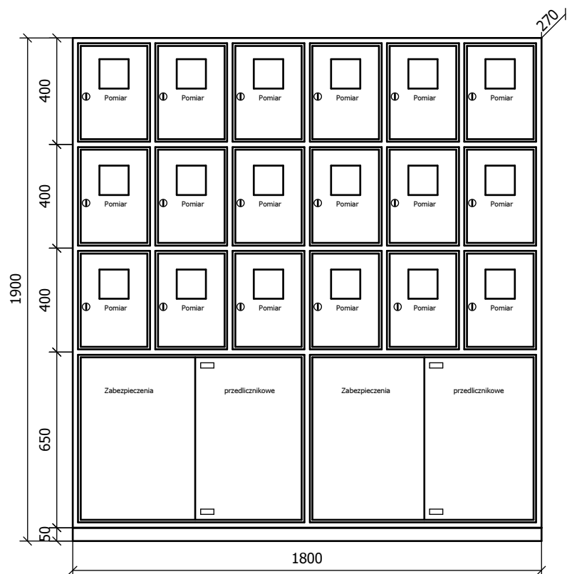
Widok elewacji
