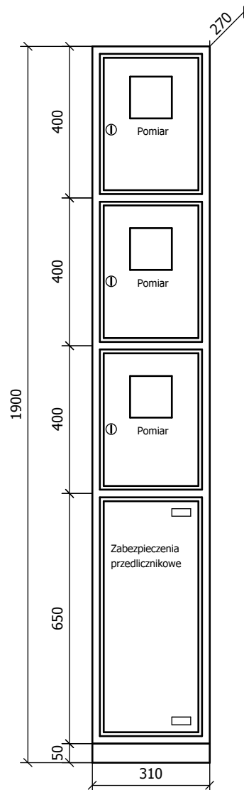
Widok elewacji
