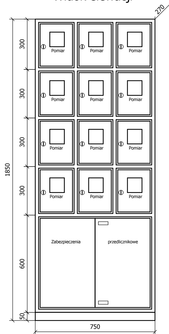
Widok elewacji
