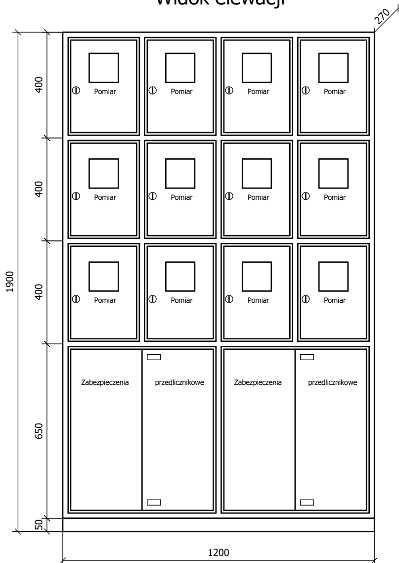
Widok elewacji
