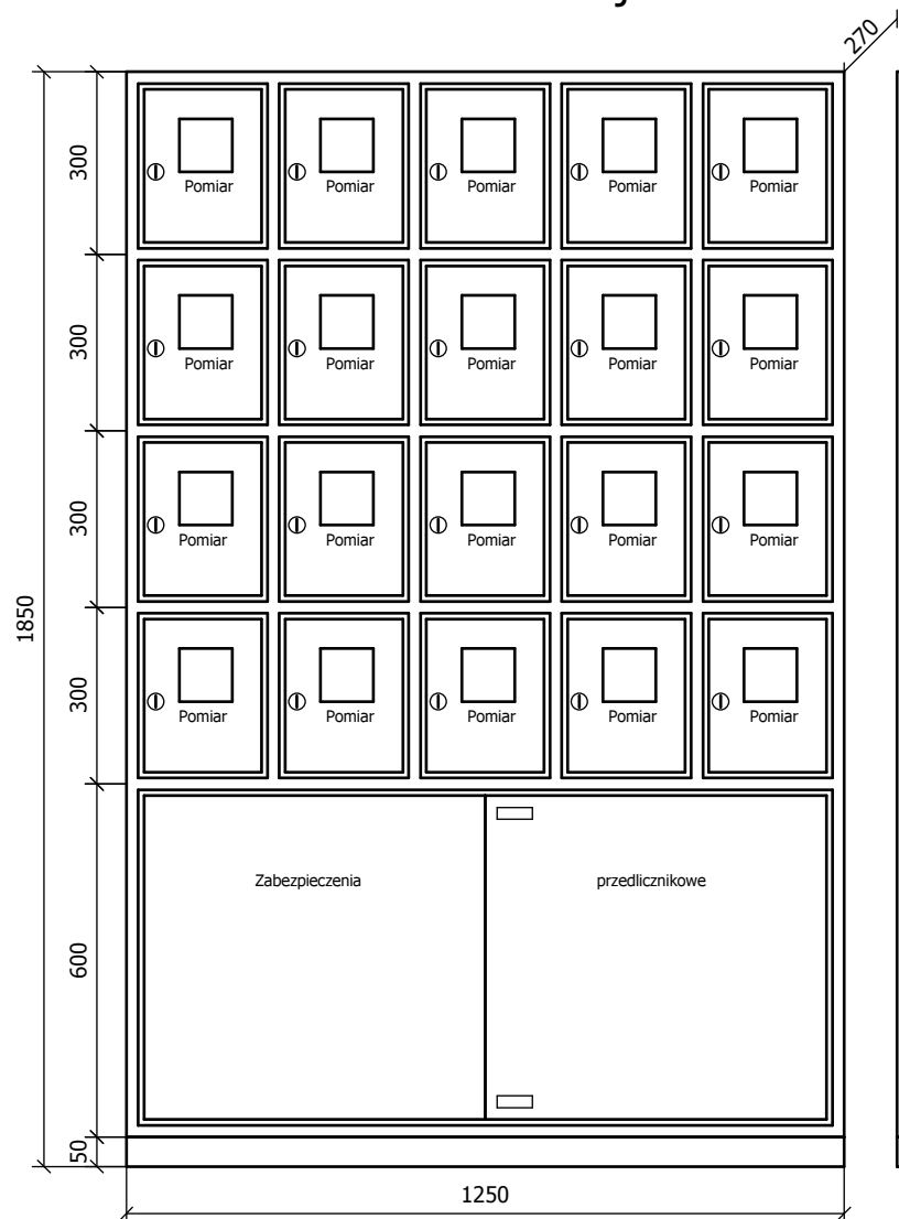
Widok elewacji
