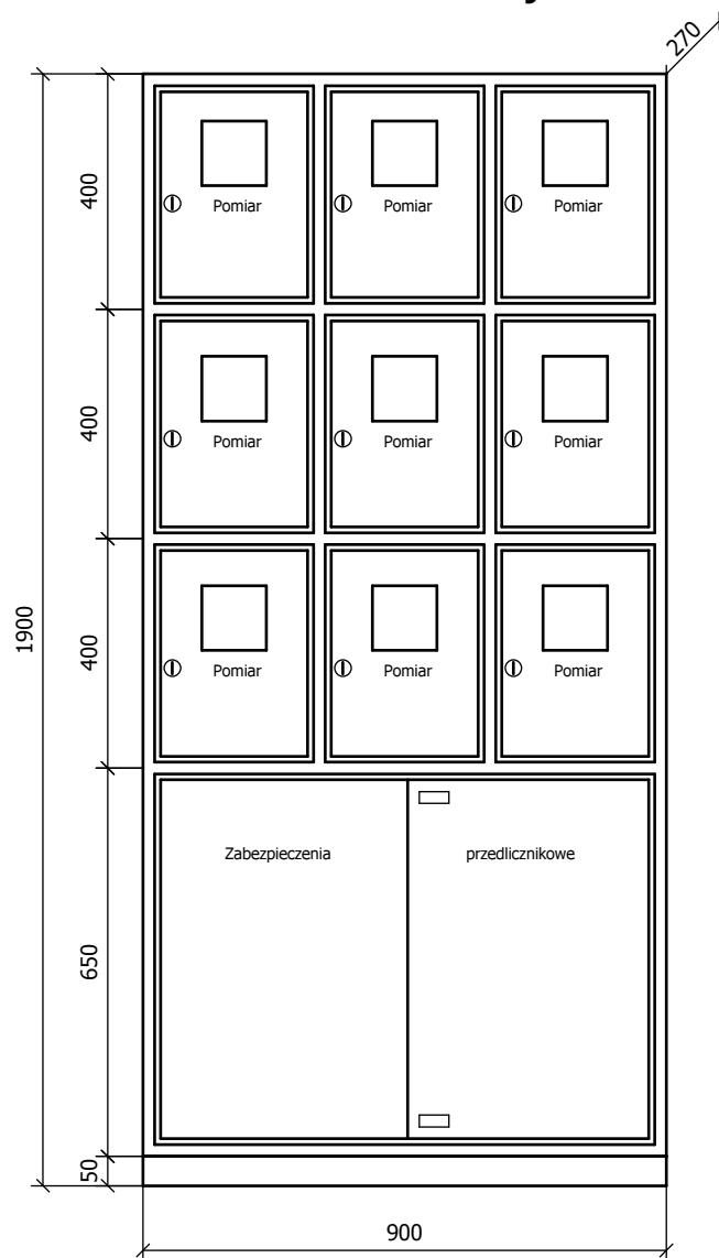
Widok elewacji
