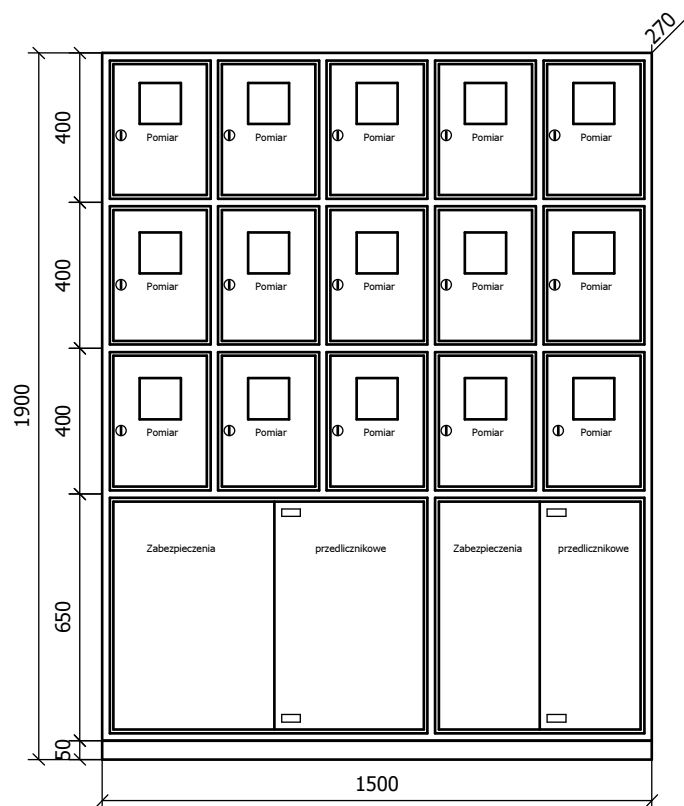
Widok elewacji
