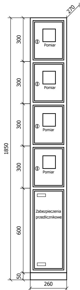
Widok elewacji
