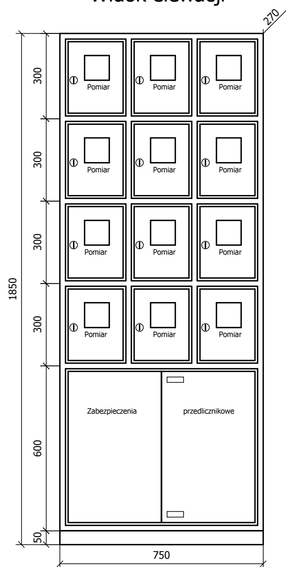
Widok elewacji
