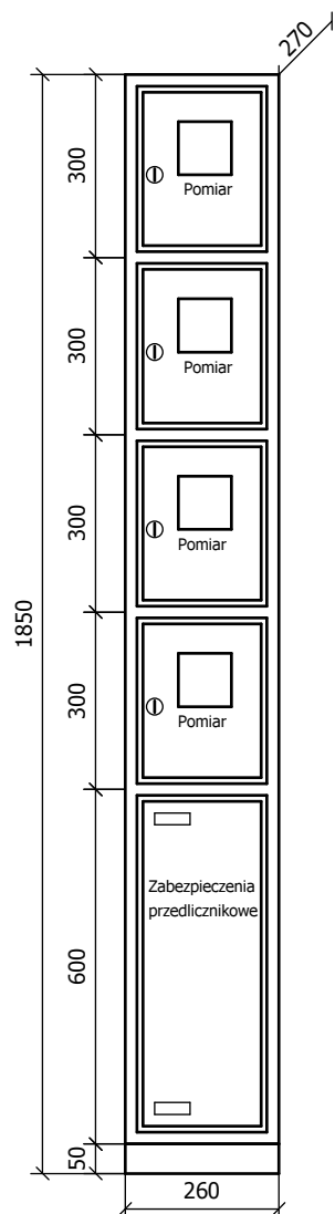
Widok elewacji
