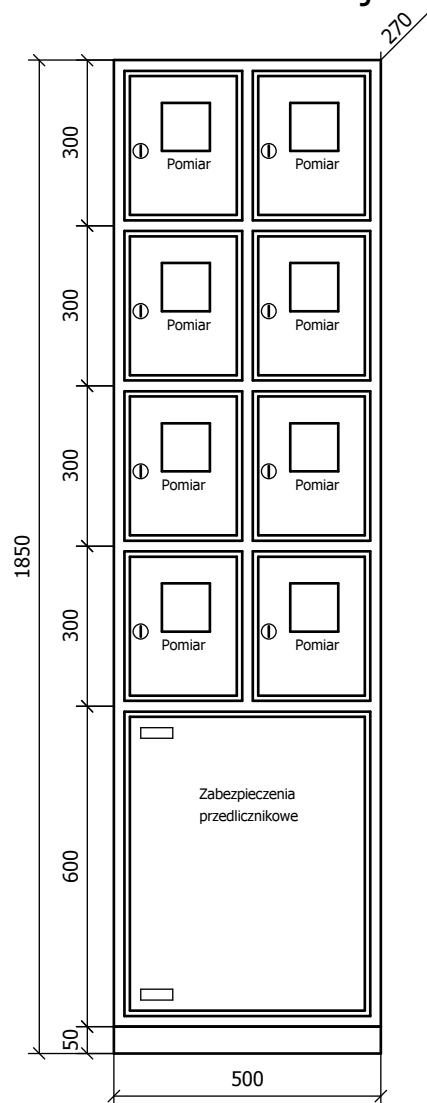
Widok elewacji
