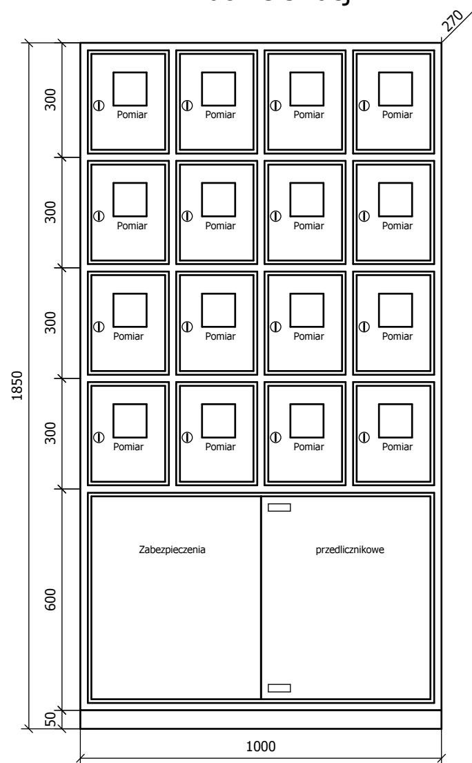
Widok elewacji
