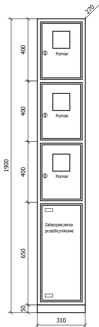
Widok elewacji
