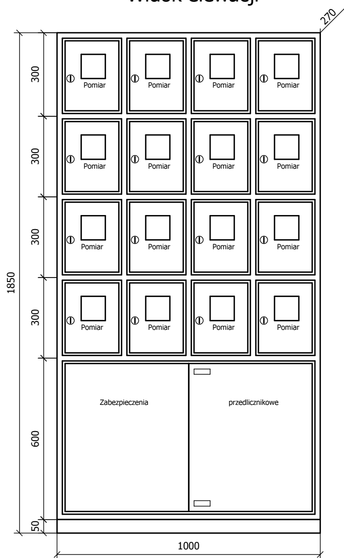
Widok elewacji
