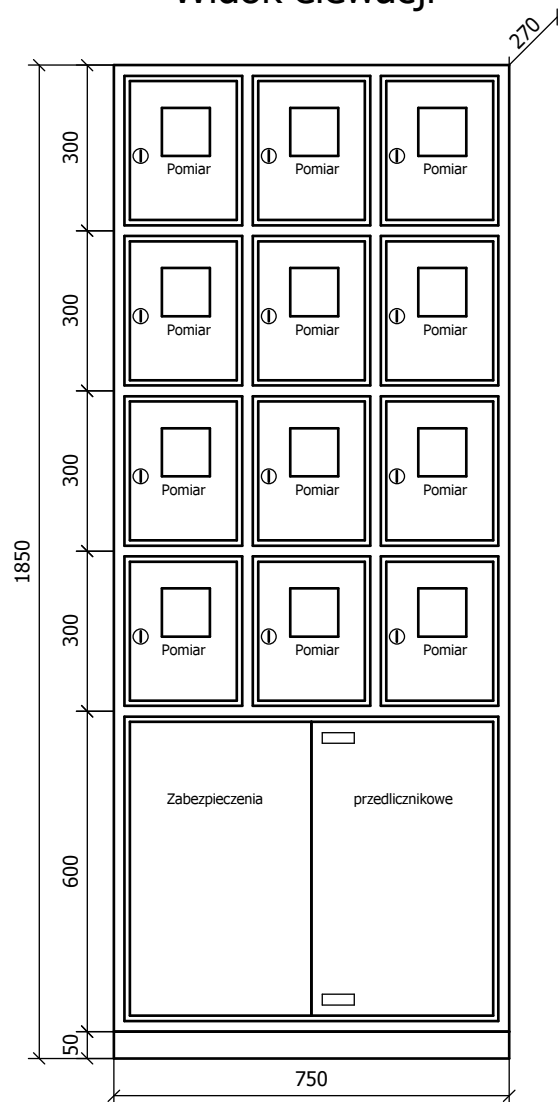
Widok elewacji
