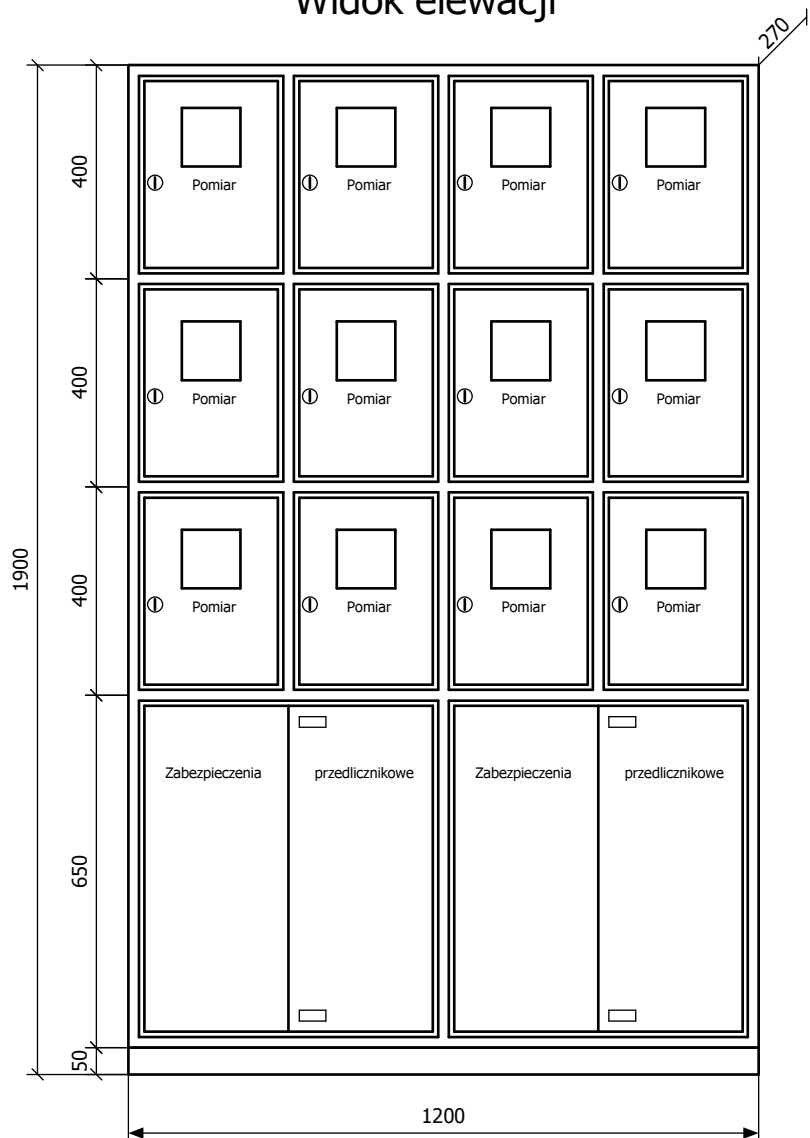
Widok elewacji
