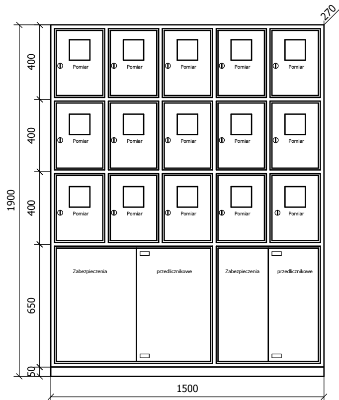
Widok elewacji
