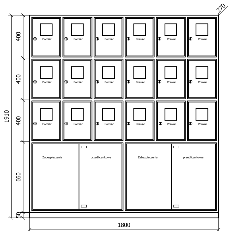
Widok elewacji
