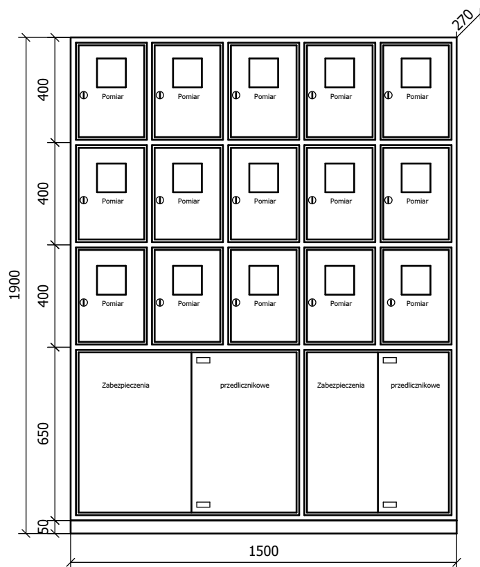
Widok elewacji
