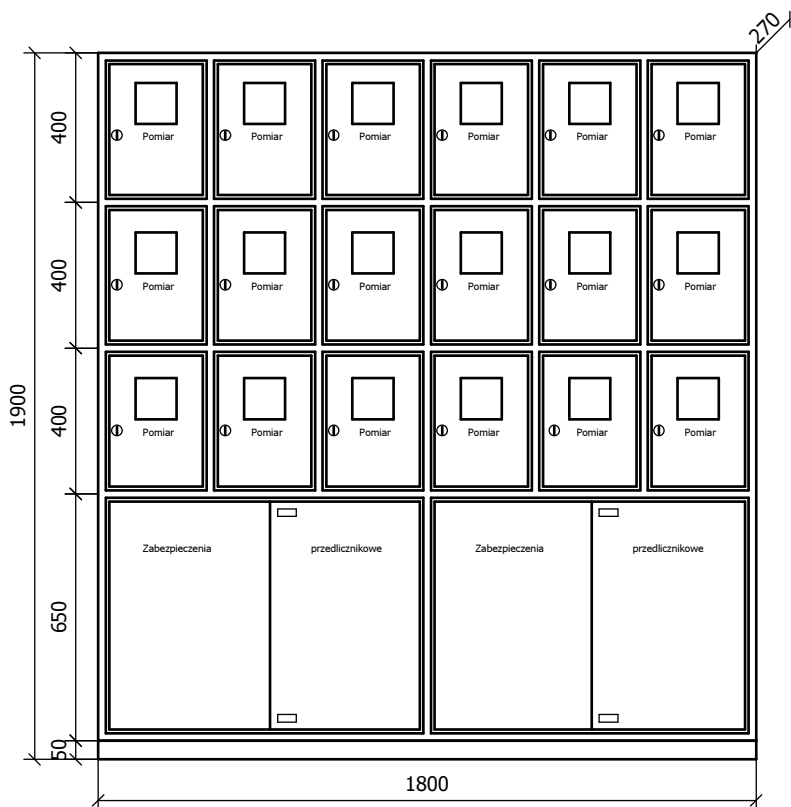
Widok elewacji
